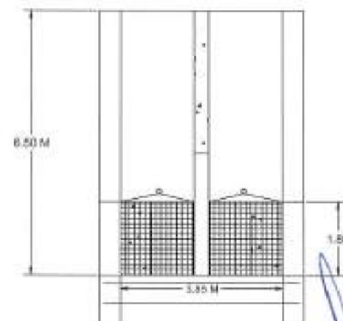
CORTE CAJA DE LLAGADA
