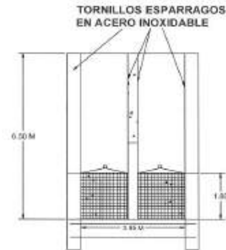
CORTE CAJA DE LLAGADA
