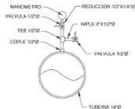
DIAGRAMA DE MEDIDOR
