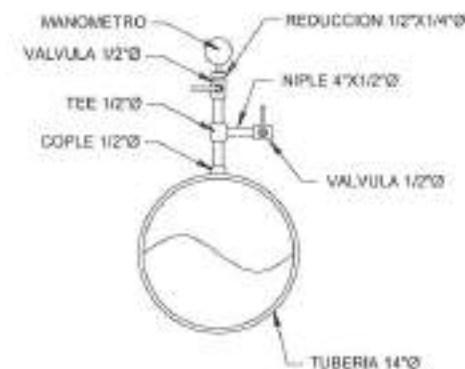
DIAGRAMA DE MEDIDOR
