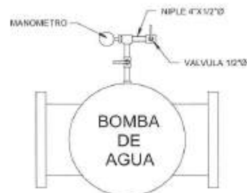
DIAGRAMA DE MEDIDOR EN BOMBA DE AGUA
