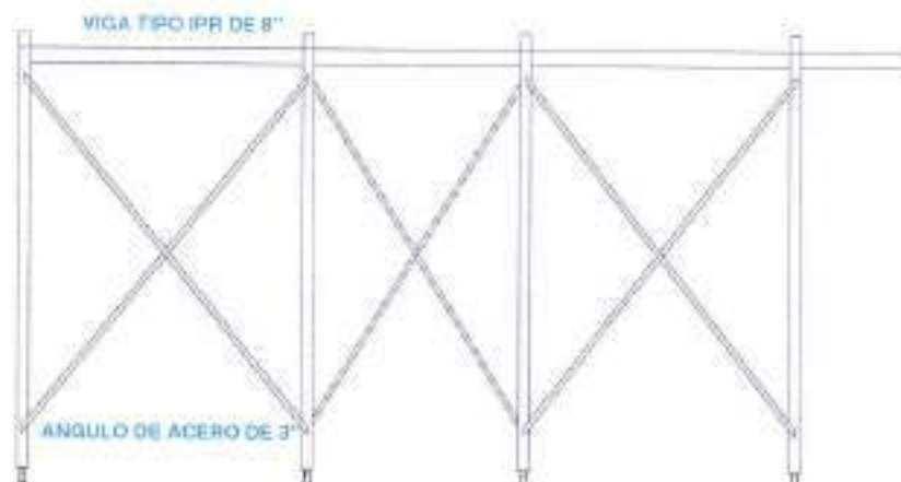
VISTA FRONTAL Estructura en CARCAMO
