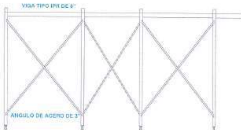
VISTA FRONTAL Estructura en CARCAMO
