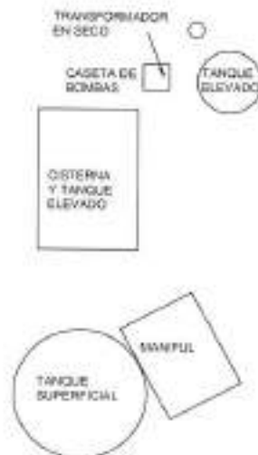
VISTA EN PLANTA REBOMBEO VILLA FLORIDA
