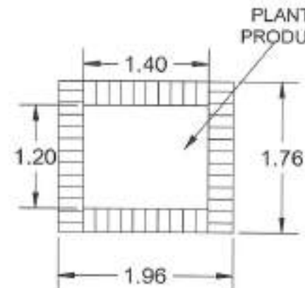
CAJA PARA OPERACION DE VALVULAS
