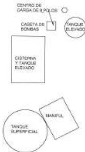
VISTA EN PLANTA REBOMBEO VILLA FLORIDA
