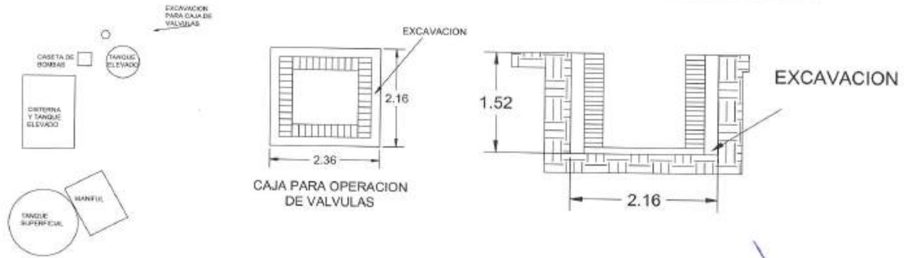
VISTA EN PLANTA REBOMBEO VILLA FLORIDA
