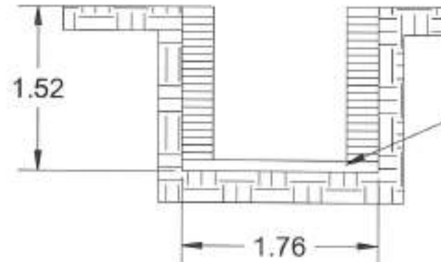
PLANTILLA DE 10 CM DE ESPESOR
