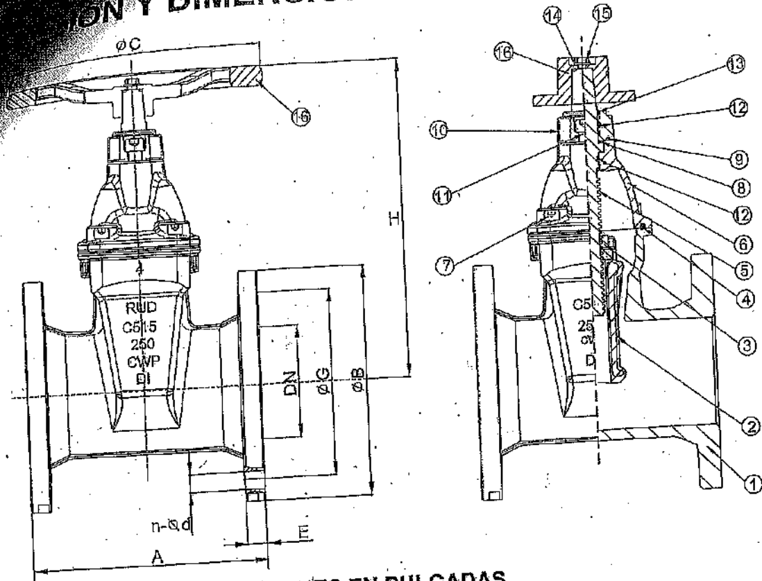
DIMENSIONES EN PULGADAS
